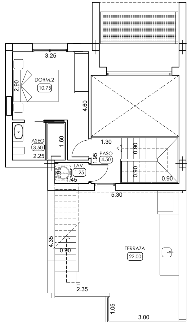
PLANTA TERCERA
