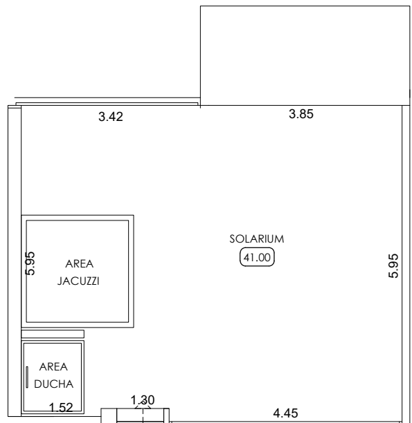
PLANTA SOLARIUM
